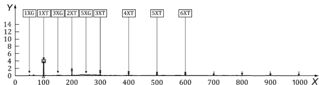
а) Вибрация в осевом направлении
