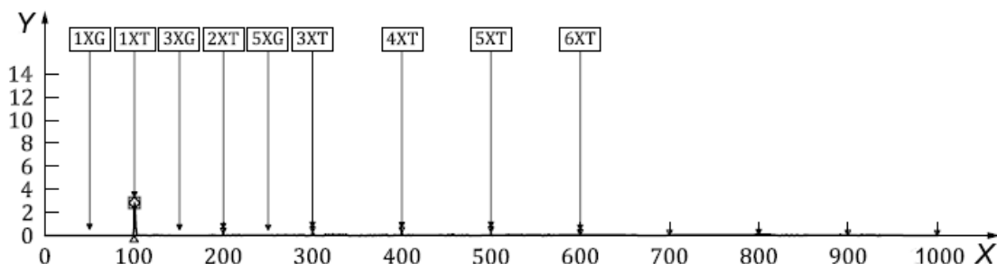
б) Вибрация в вертикальном направлении
