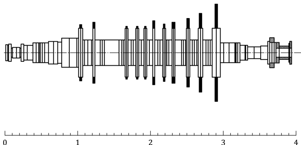
Рисунок С.3 – Схема турбины
