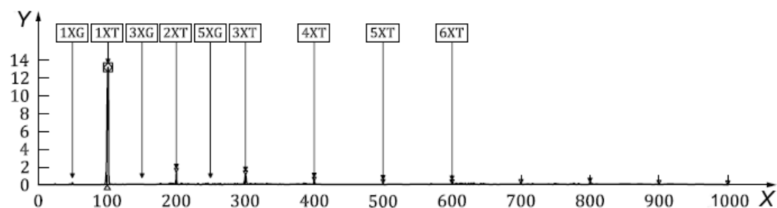
в) Вибрация в горизонтальном направлении
