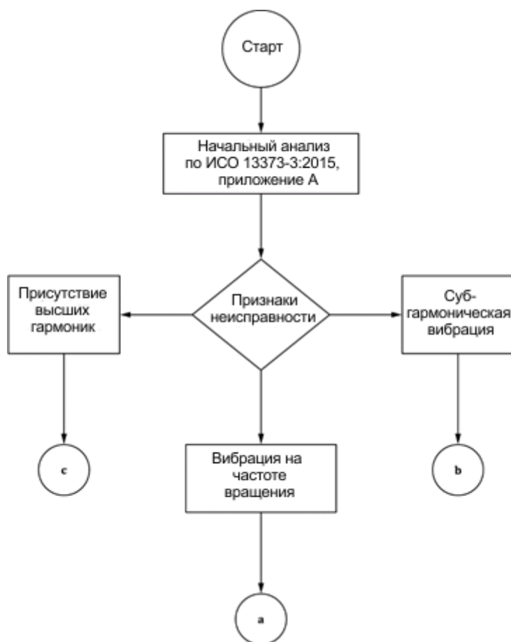
Рисунок В.1 – Схема вибрационного диагностирования газовых и паровых турбин с гидравлическими подшипниками
