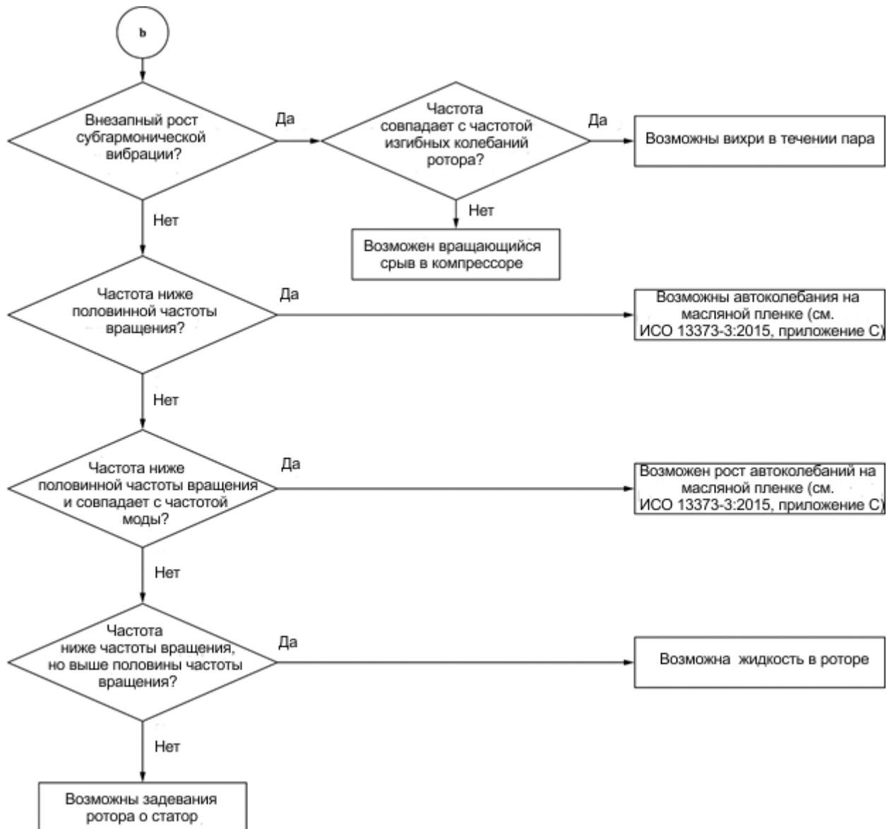
Рисунок В.3 – Схема диагностирования газовых и паровых турбин с гидравлическими подшипниками при наличии вибрации в области субгармонических частот
